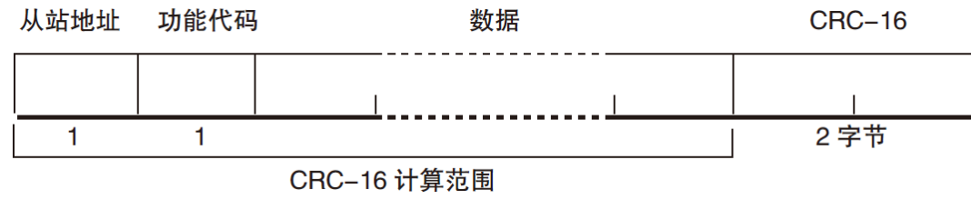
图 11-3 正常响应帧
