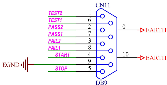
图 4-6 DB9 针形 Handler 插头接线柱
