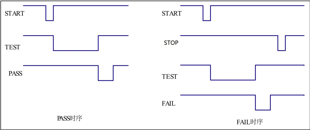
图 8-3 PLC 时序图
