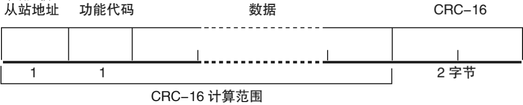
图 10-4 异常响应帧
