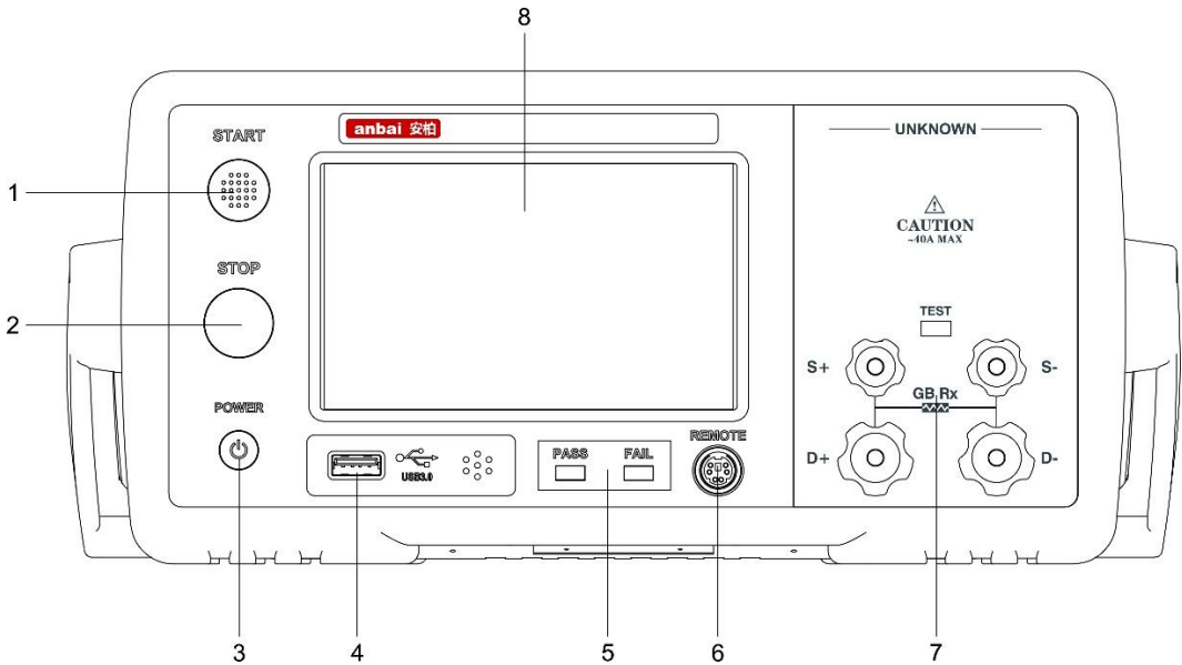
图 3-1 AT9600 前面板
