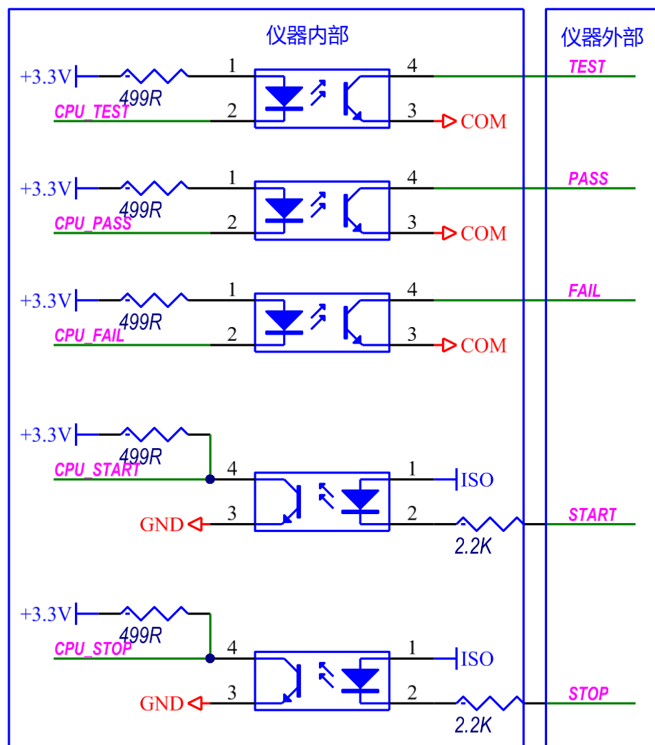
图 7-2 仪器 Handler 接口内部电路结构
