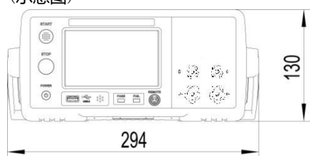
图 n-n 外形 (示意图)
