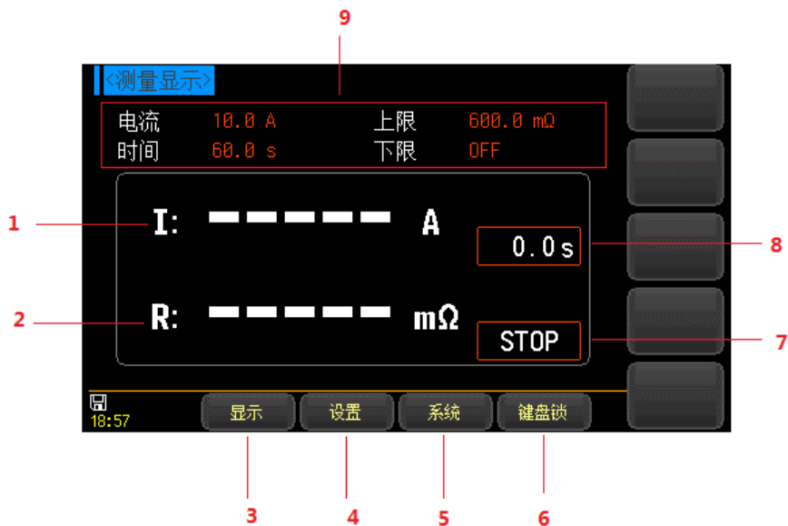
图 5-1 <测量显示> 页
