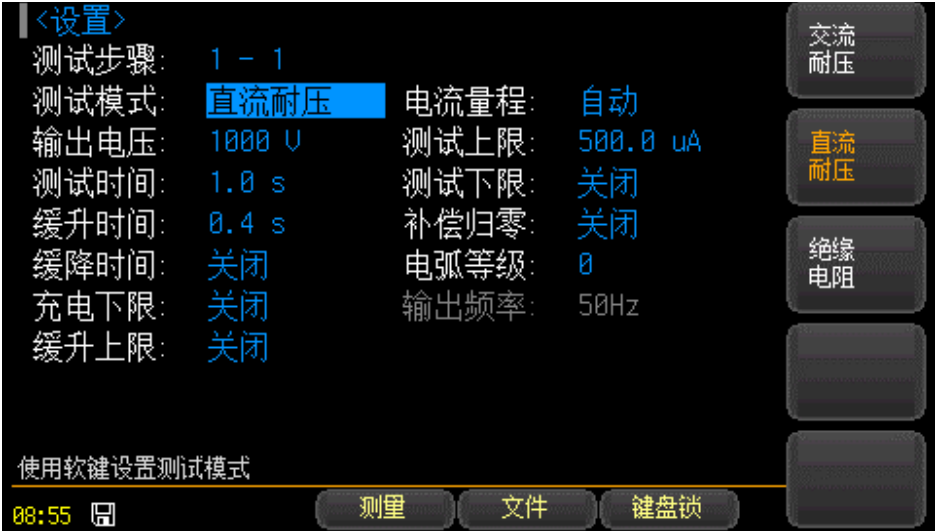
图 5-3 【直流耐压】设置
