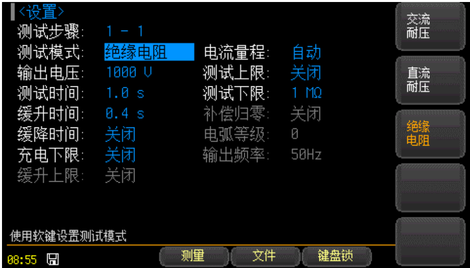
图 5-4 【绝缘电阻】设置
