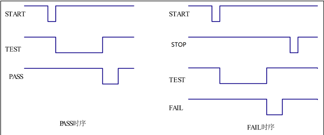
图 8-4 PLC 时序图
