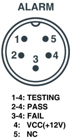
图 8-1 报警灯接口插座（公）
