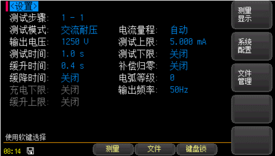
图 5-2 【交流耐压】设置
