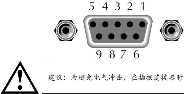
图 9-1 后面板上 RS-232 接口
