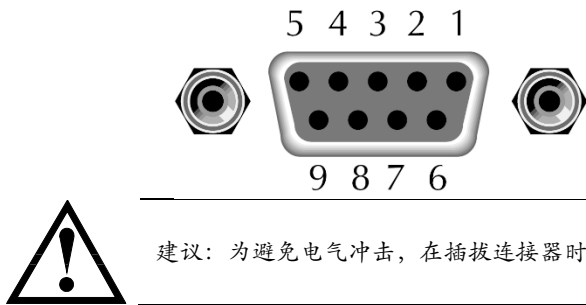
图 9-1 后面板上 RS-232 接口
