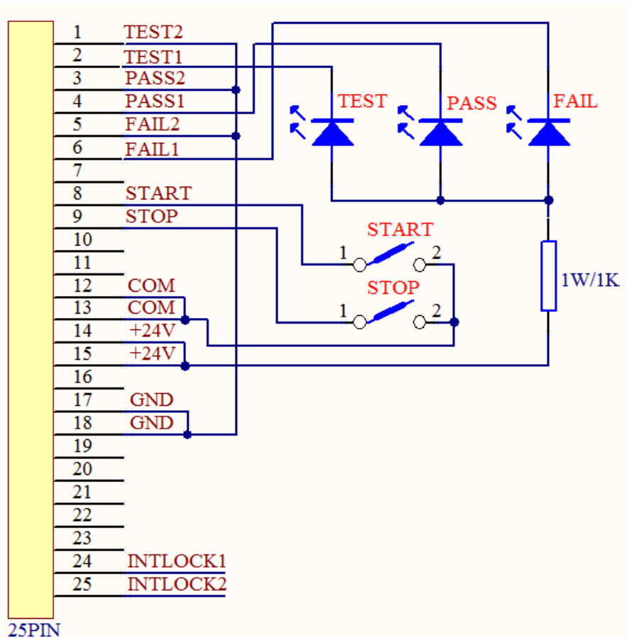
仪器接口外部连接
