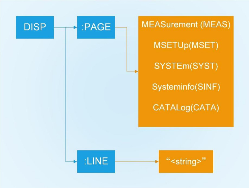
图 10-2 DISPlay 子系统树 DISPlay 子系统可以用来切换不同的显示页面或在页面提示栏上显示一串文本。
