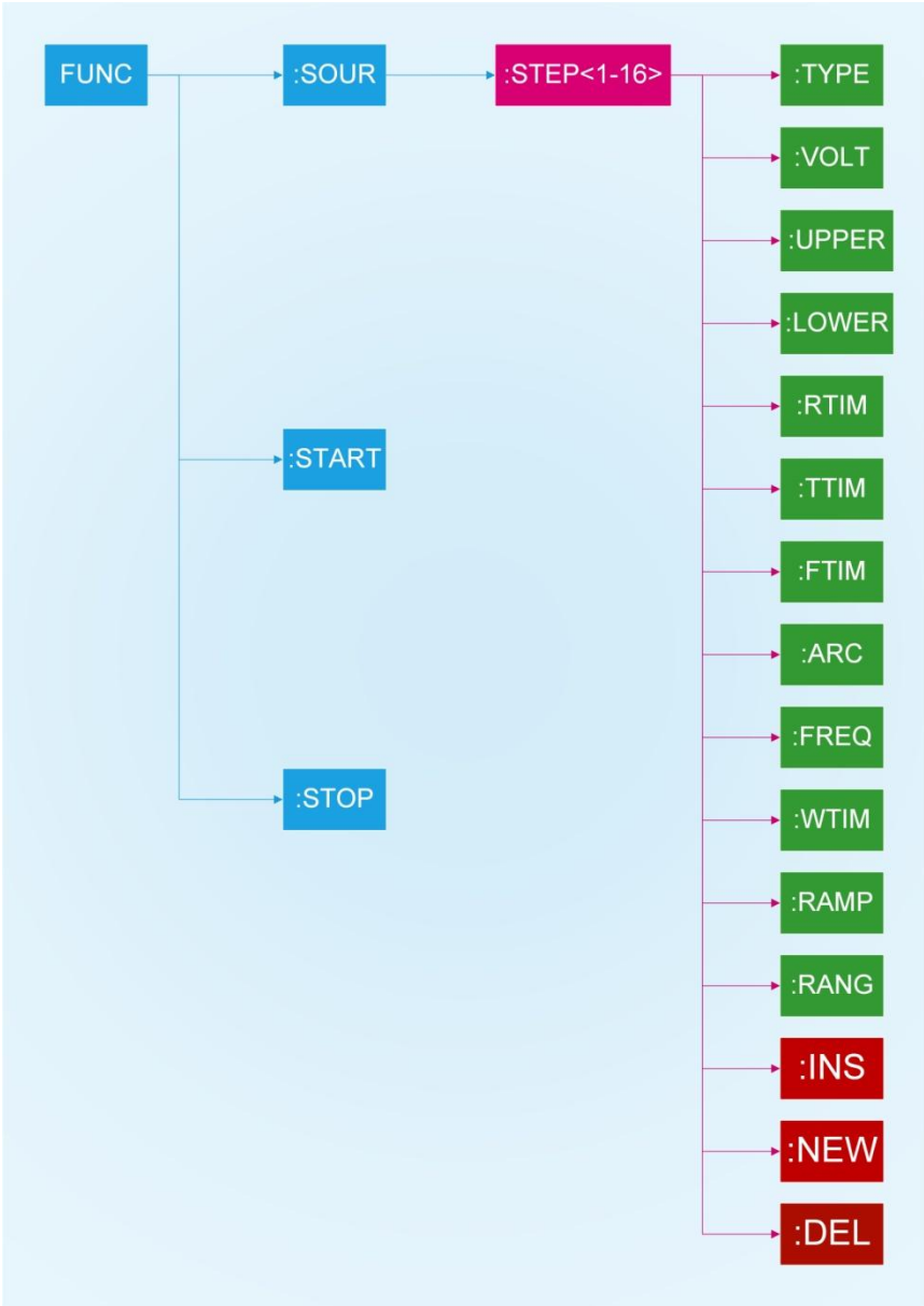
图 10-11-3 FUNCTION 子系统树
