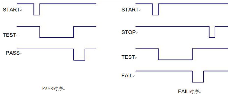
图 9-3 仪器 Handler 接口默认测试时序
