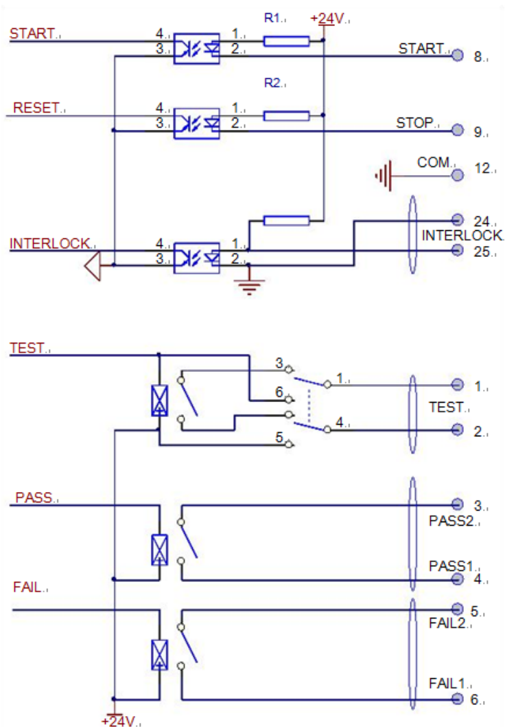
图 9-2 仪器 Handler 接口内部电路结构
