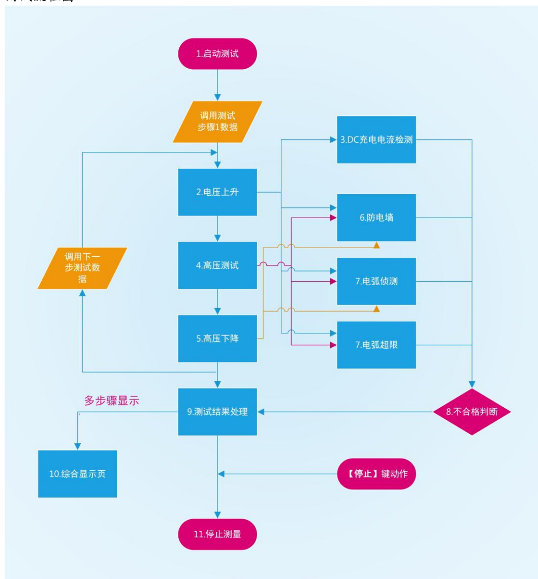
图 5-2 测试流程图
