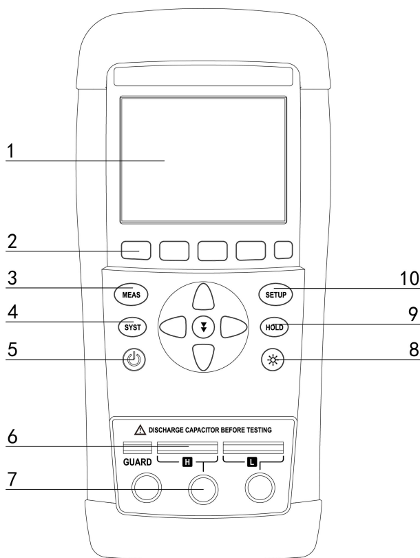
图 3-1 前面板
