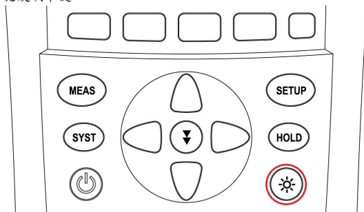
图 6-2 亮度调节键
