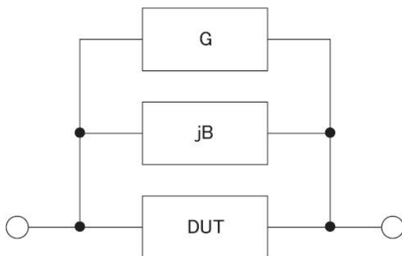
图 5-3 杂散导纳
