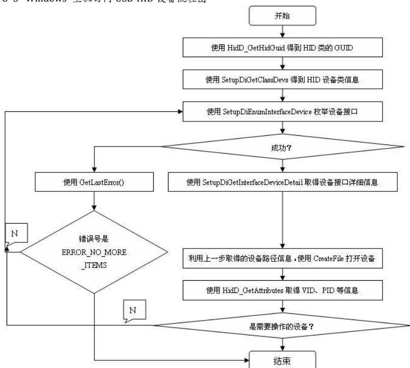
图 8-3 Windows 主机访问 USB-HID 设备流程图
