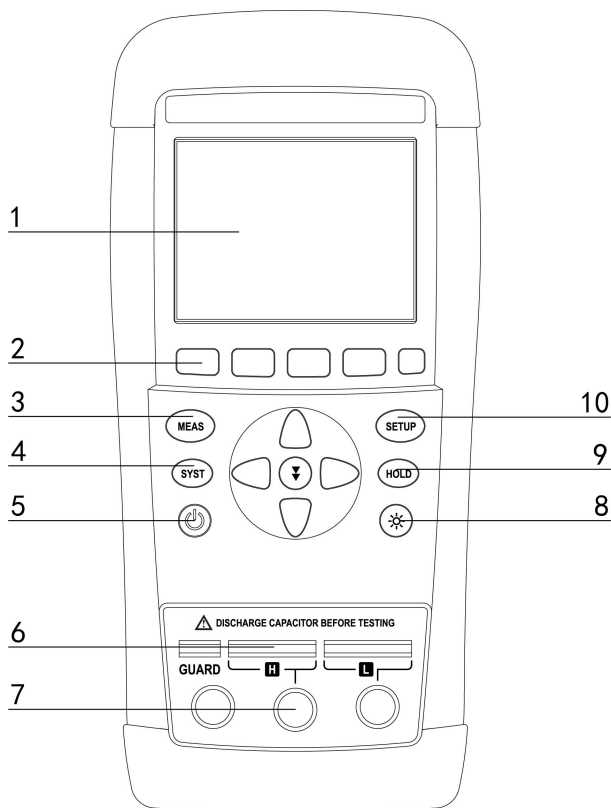
图 3-1 前面板
