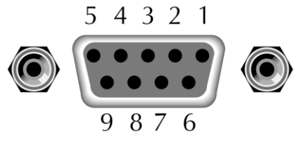
图 9-1 后面板上 RS-232 接口
