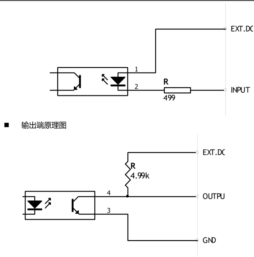
图 4-2 内部原理图
