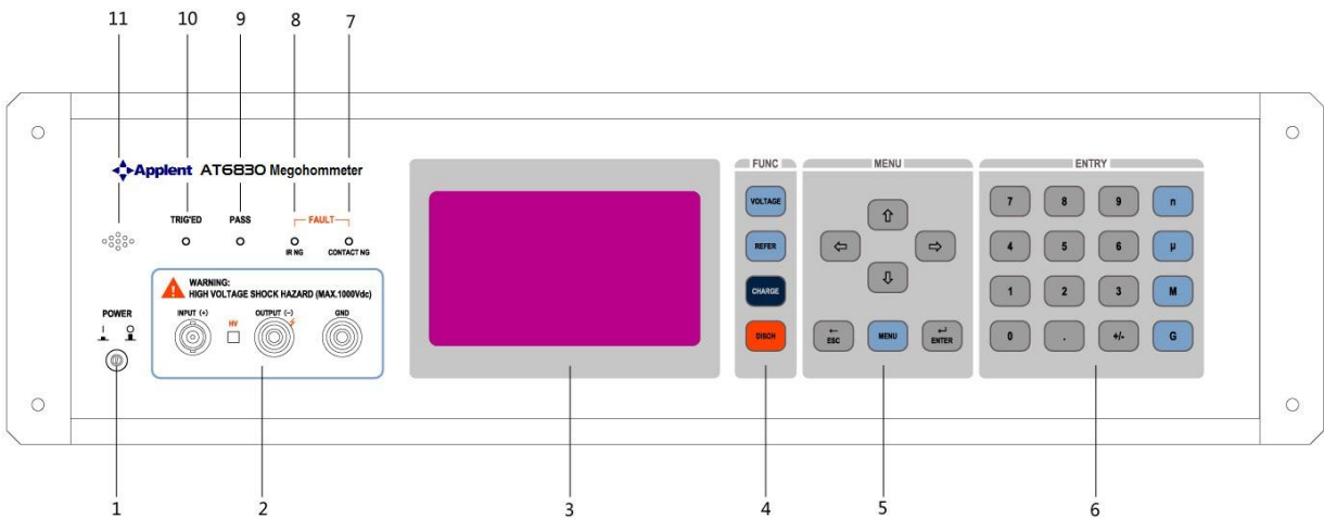
图 3-1 前面板
