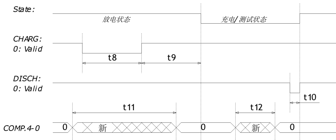
图 4-3 周期表
