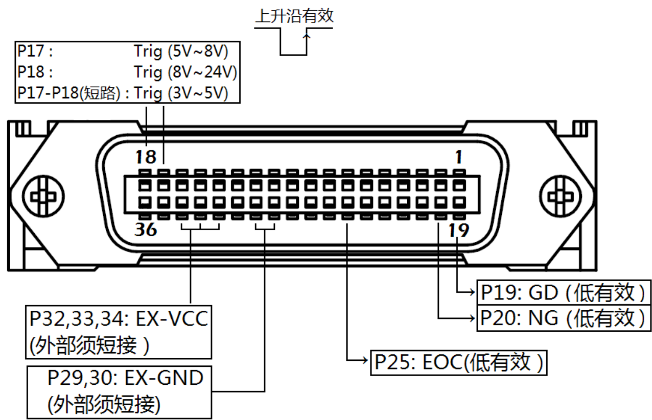
图 4-1 接线端子
