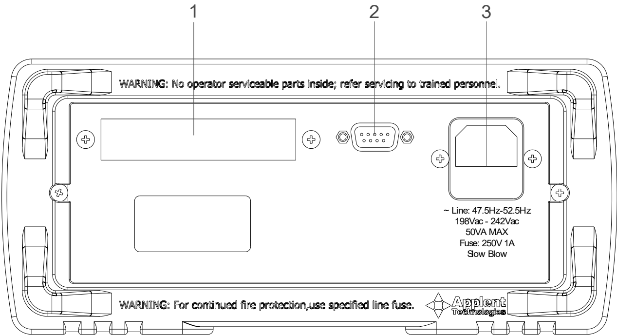
图 3-5 后面板
