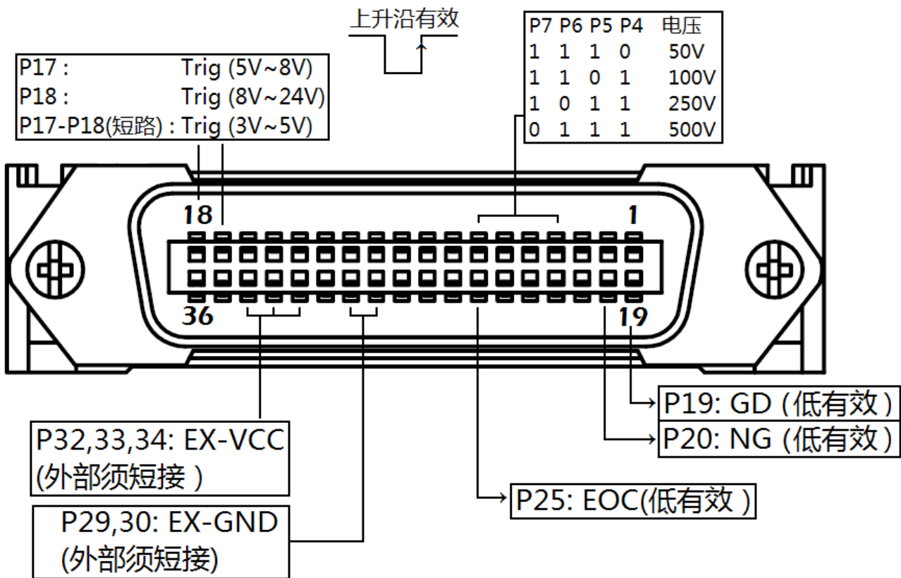
图 4-1 接线端子
