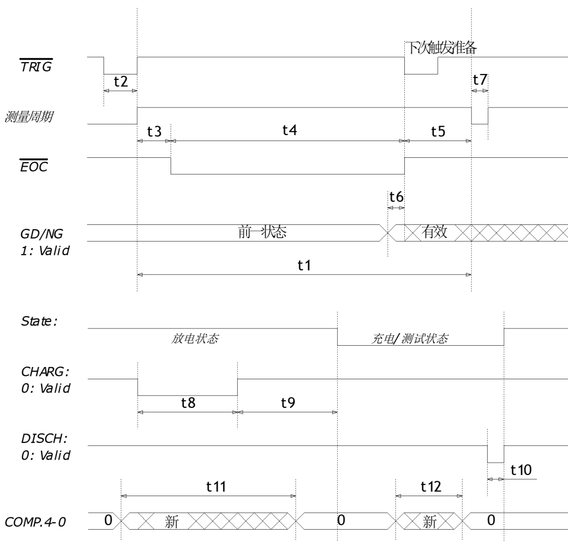
图 4-3 周期表
