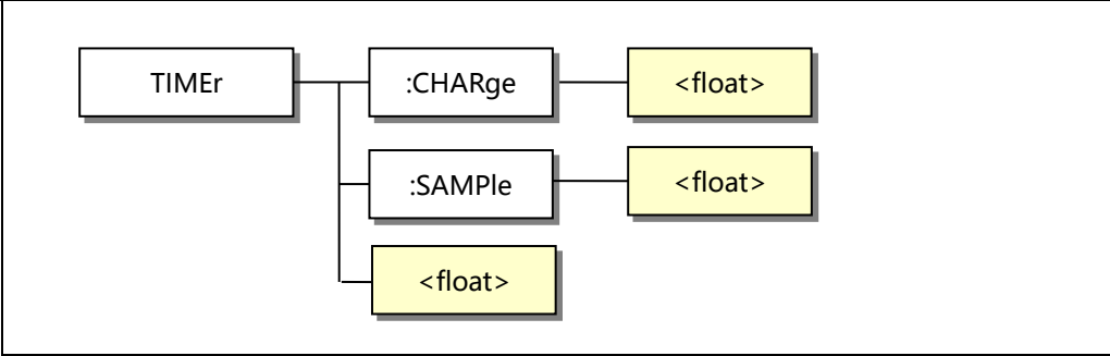
图 6-7 TIMEr 命令树
