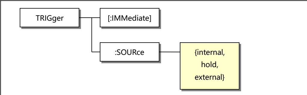
图 6-10 TRIGger 命令树
