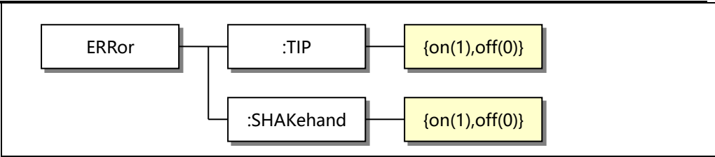
图 6-12 ERRor? 命令树
