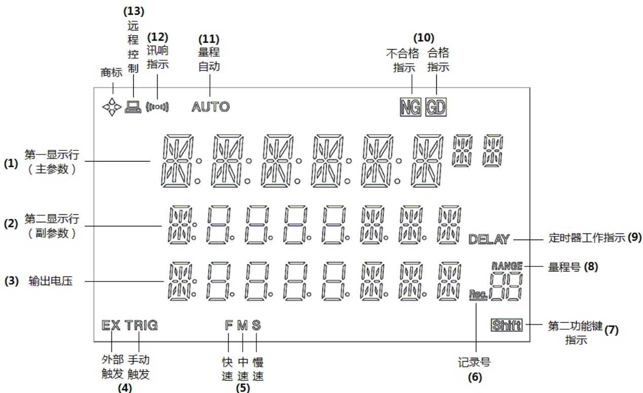
图 3-2 显示屏
