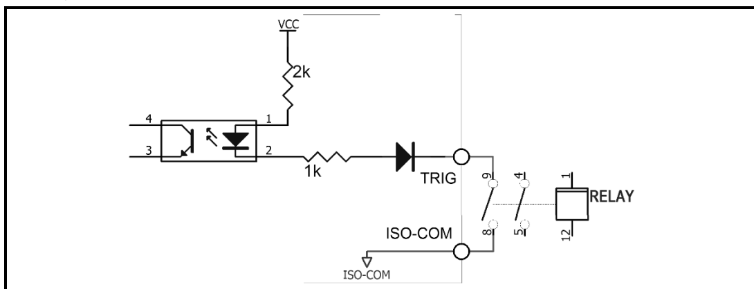
图 12-5 使用继电器控制
