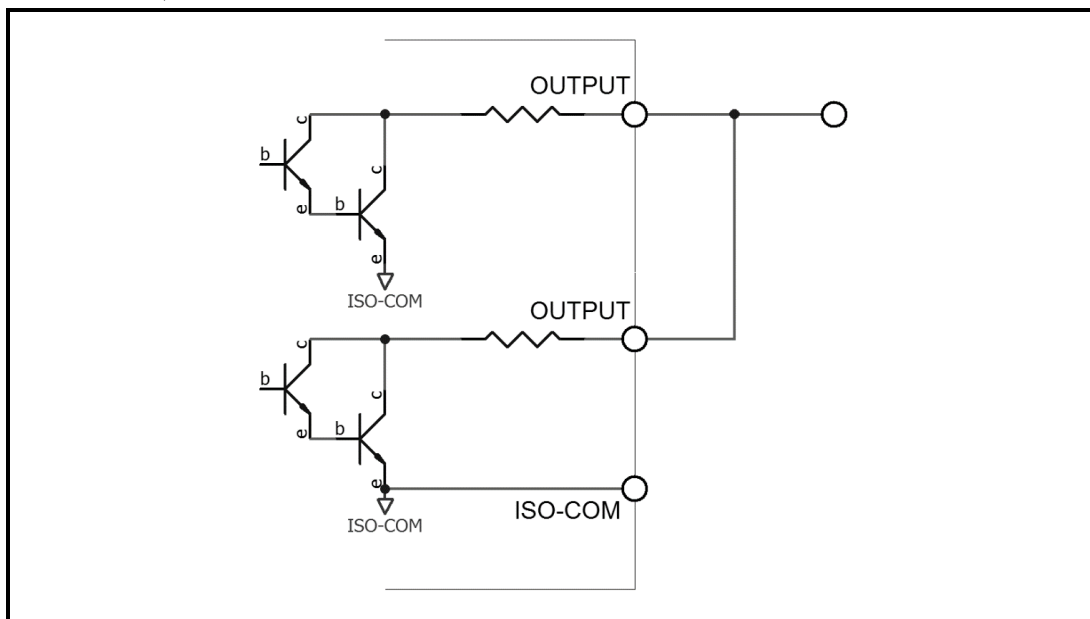
图 12-11 双端口输出组成逻辑或电路
