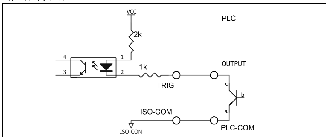
图 12-6 使用 PLC 负公共端子控制
