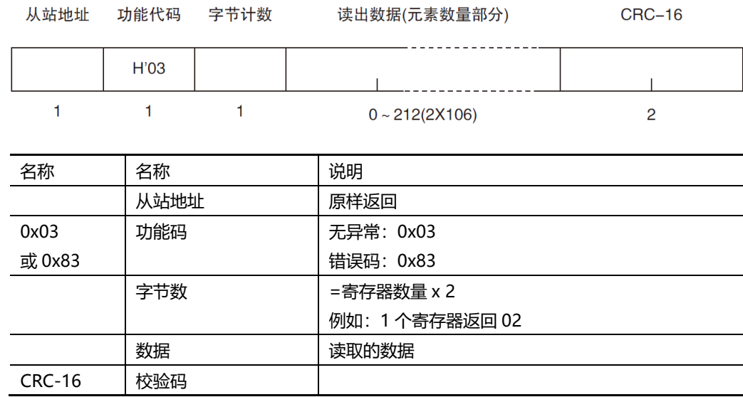
图 15-6 读出多个寄存器 (0x03) 响应帧
