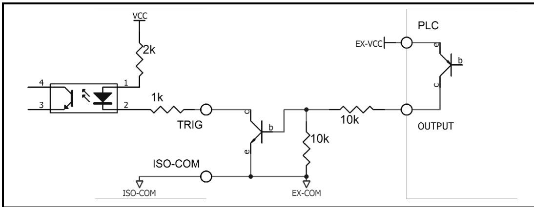
图 12-7 使用 PLC 正公共端子控制
