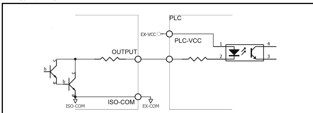
图 12-12 输出到 PLC 负公共端子
