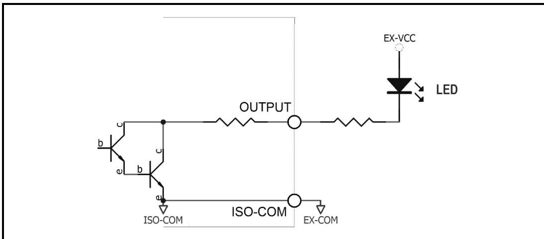
图 12-9 控制发光二极管或光电耦合器
