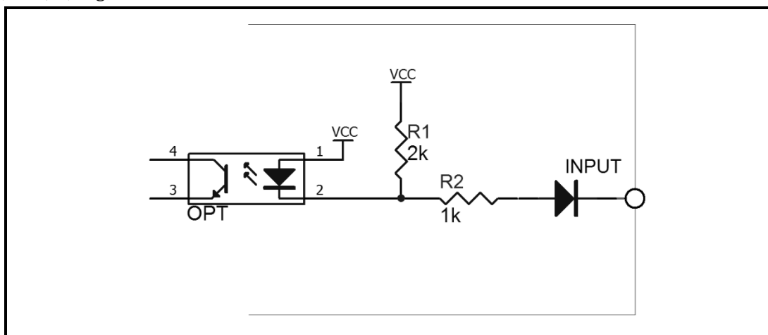
图 12-2 输入端原理图 (Trig)
