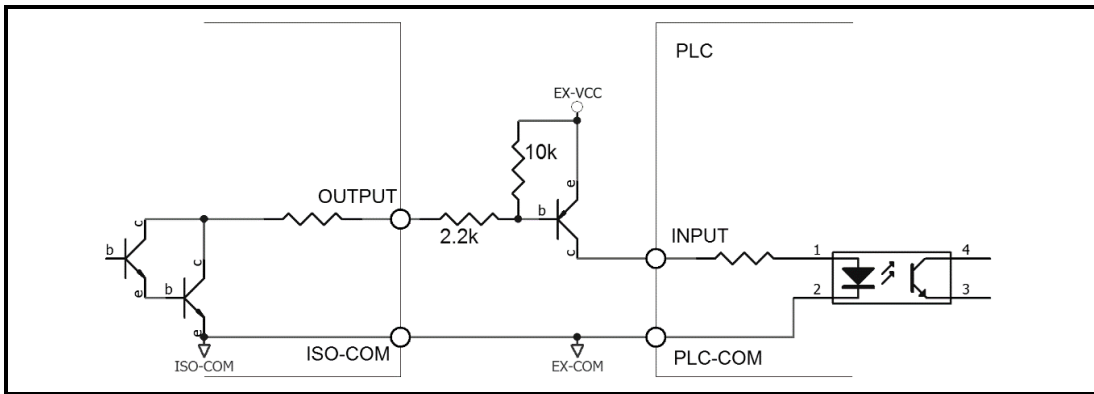
图 12-13 输出到 PLC 正公共端子
