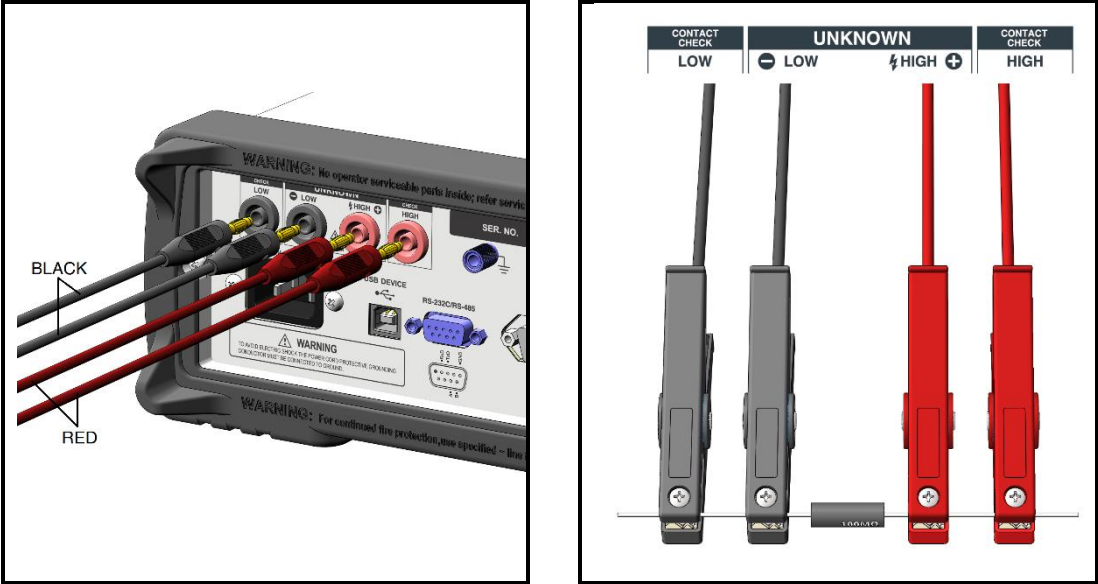
图 5-2 后面板接触不良端子连接
