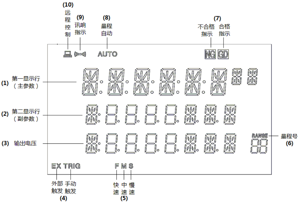
图 3-2 显示屏幕
