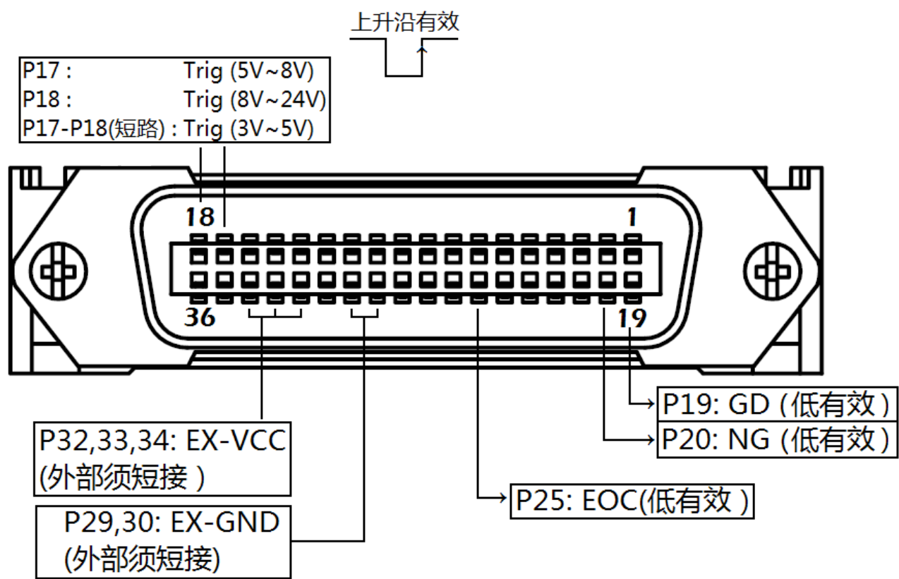
图 4-1 接线端子
