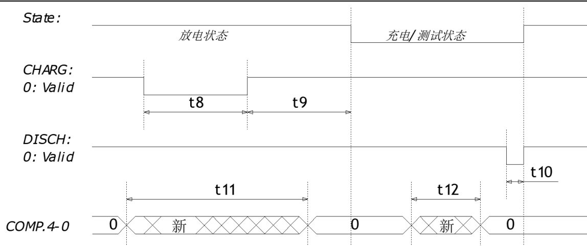
图 5-4 周期表
