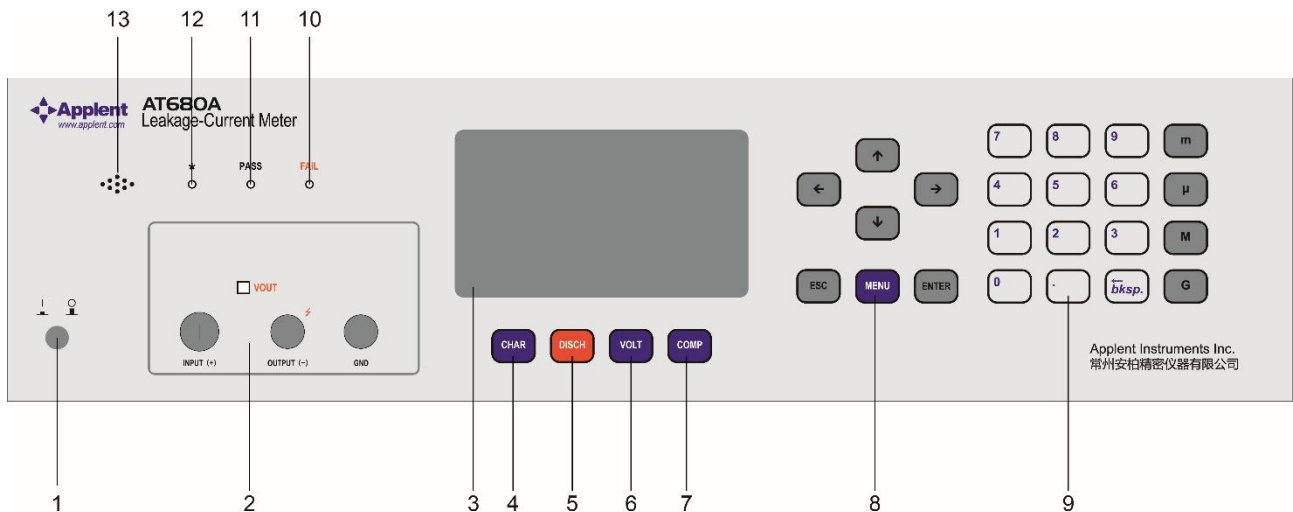
图 3-1 前面板
