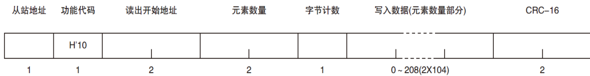
图 9-7-6 写入多个寄存器 (0x10)
