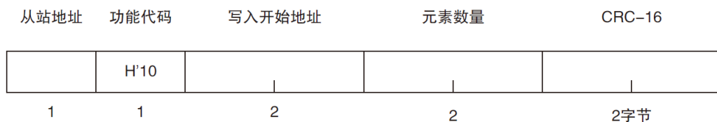
图 9-7-7 写入多个寄存器 (0x03) 响应帧
