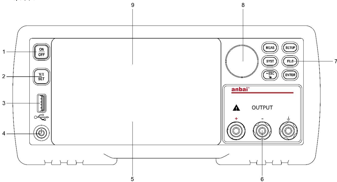
图 3-1 前面板
