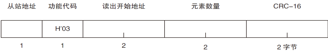
图 9-7-4 读出多个寄存器（0x03）
