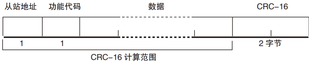
图 9-3 异常响应帧
