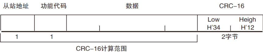
图 11-2 Modbus 附加 CRC-16 值
