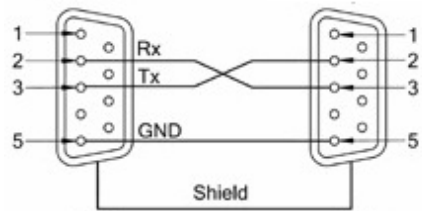
图 9-2 后面板上 RS-232 接口[公头]
