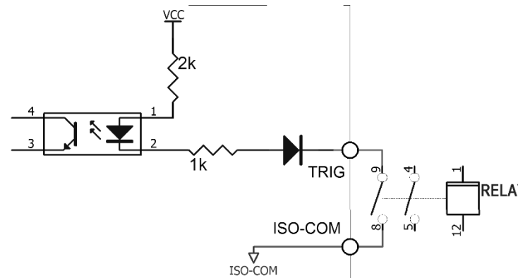
图 8-6 使用 PLC 负公共端子控制
