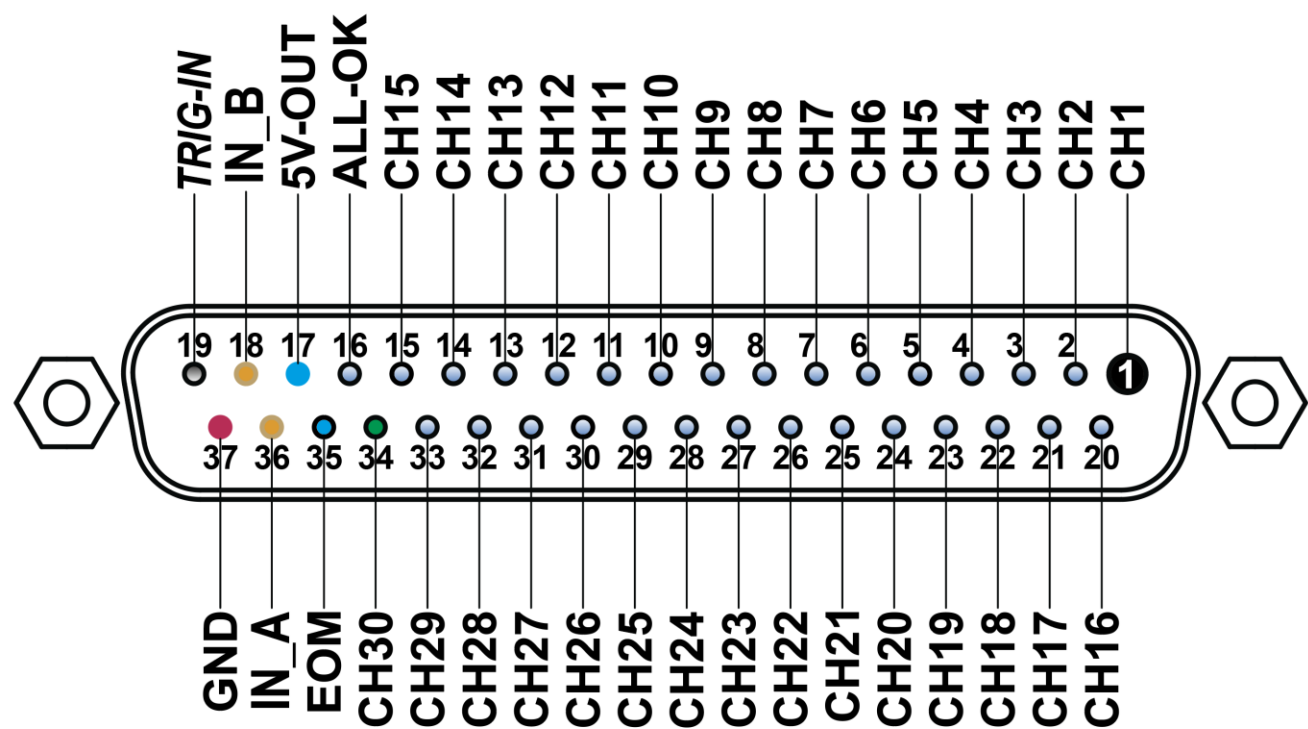
图 8-1 接线端子
