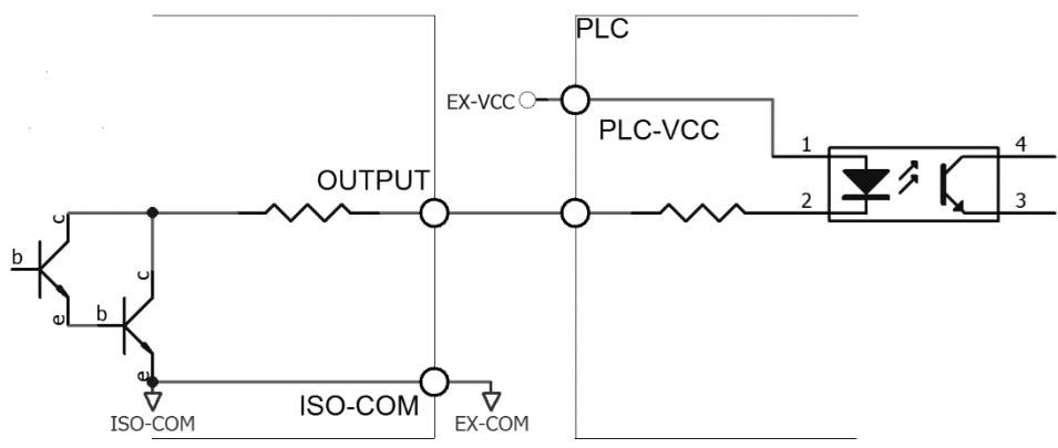
图 8-13 输出到 PLC 正公共端子
