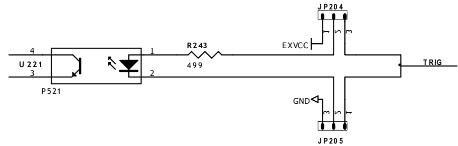
图 7-2 输入端原理图（Trig）
