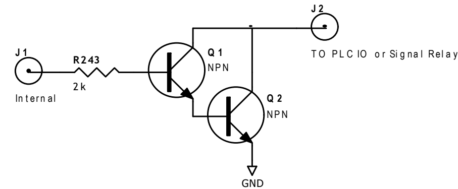
图 7-3 输出端原理图
