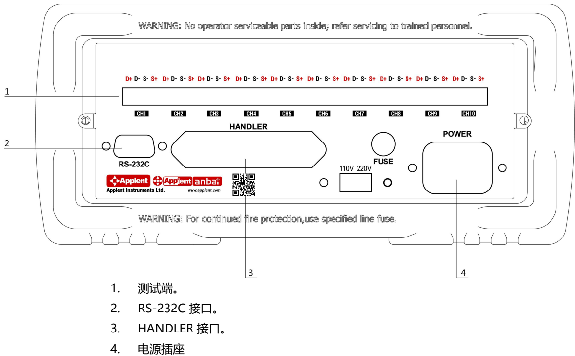
图 3-2 后面板
