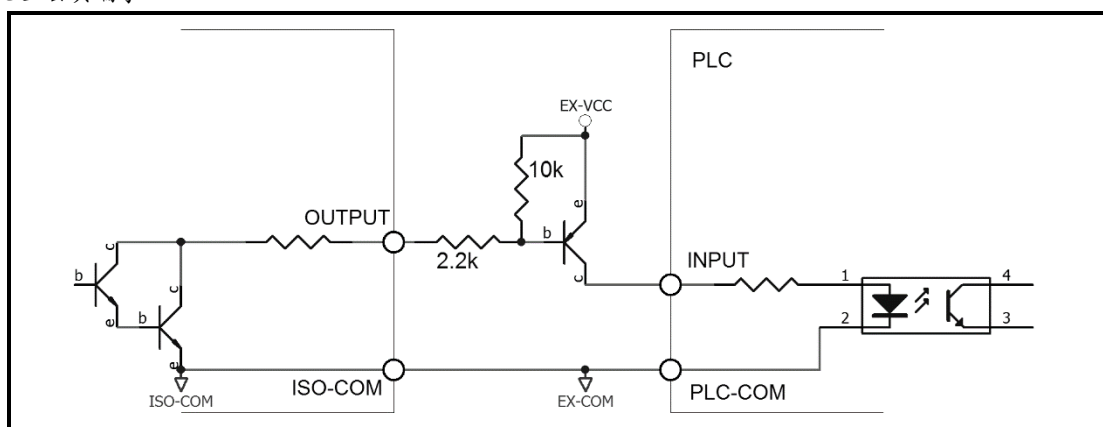
图 9-13 输出到 PLC 正公共端子
