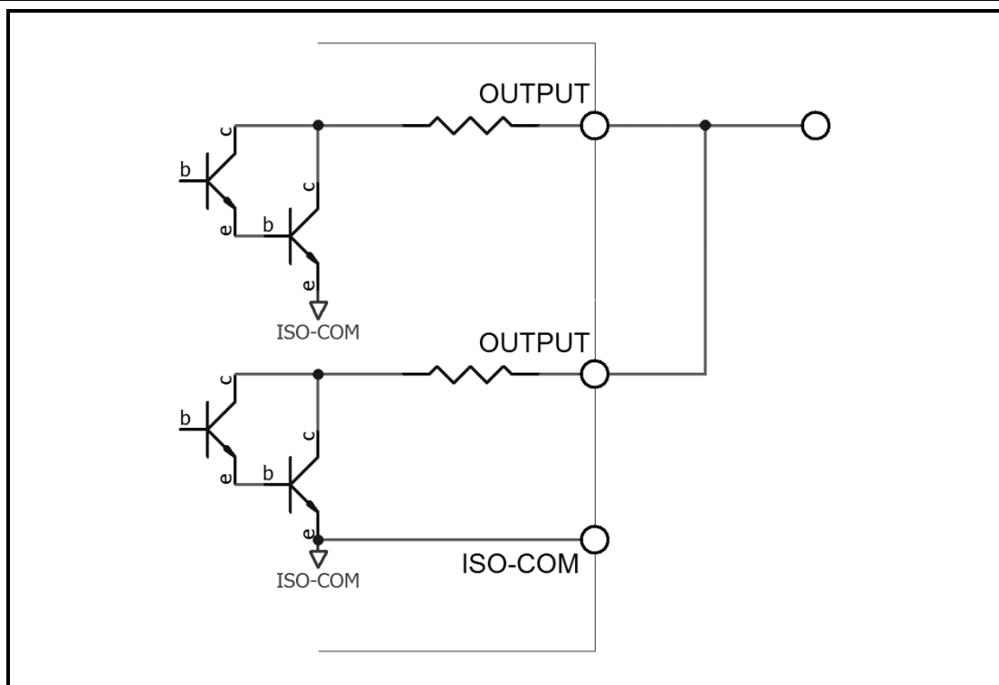
图 9-12 输出到 PLC 负公共端子
