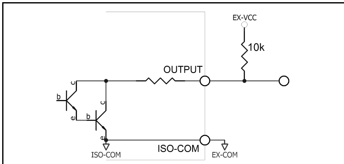
图 9-11 双端口输出组成逻辑或电路
