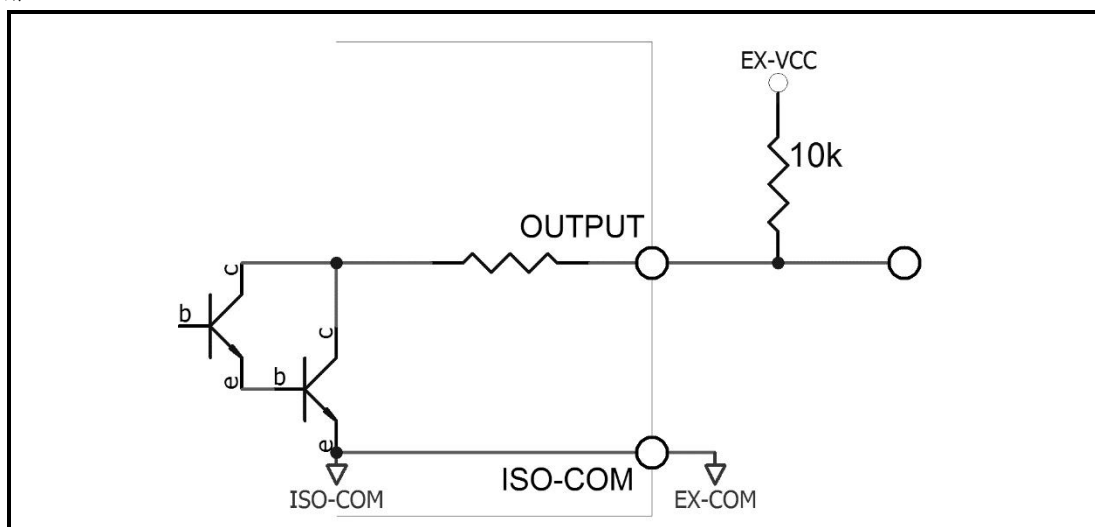
图 7-11 双端口输出组成逻辑或电路
