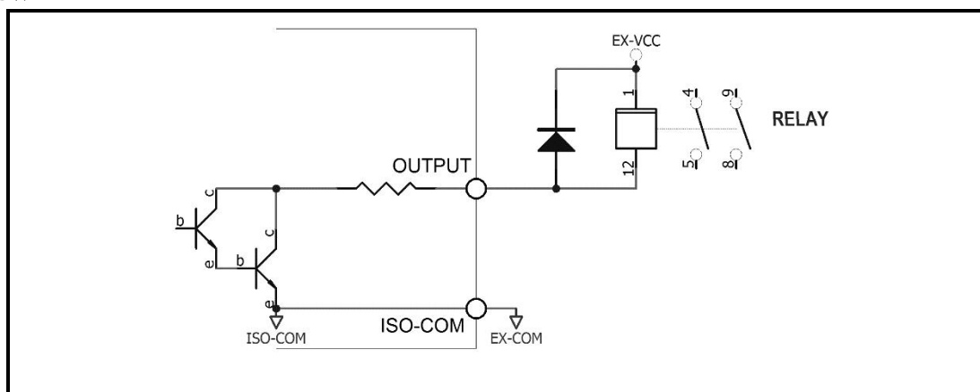
图 7-9 控制发光二极管或光电耦合器
