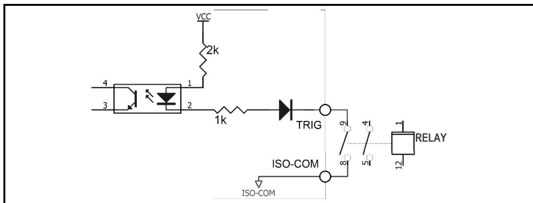
图 7-5 使用继电器控制
