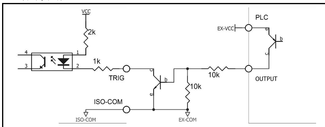
图 7-7 使用 PLC 正公共端子控制
