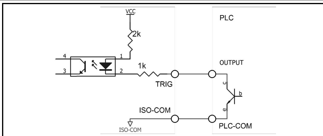
图 7-7 使用 PLC 正公共端子控制
