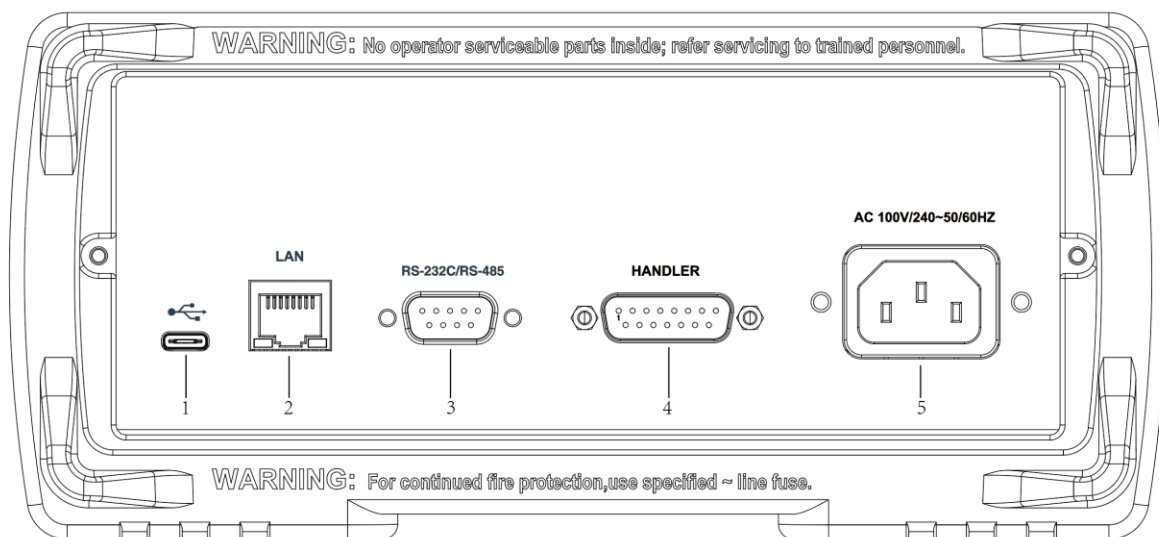
图 3-2 后面板
