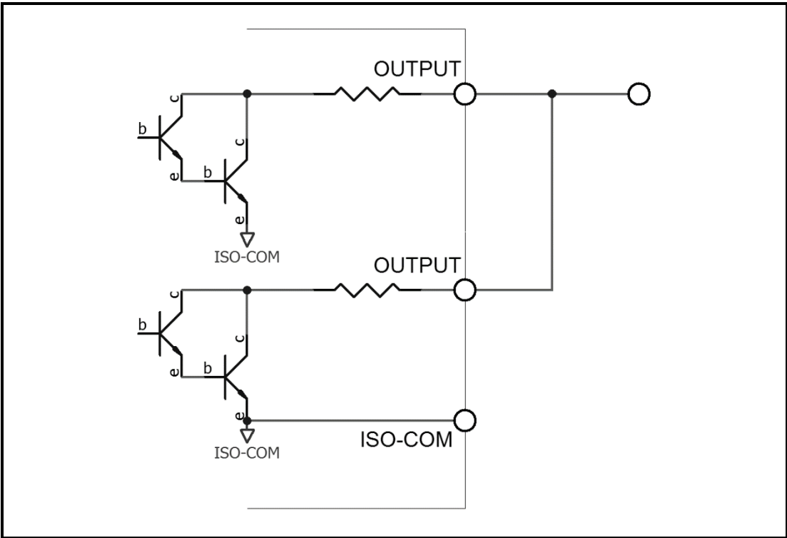
图 8-12 输出到 PLC 负公共端子
