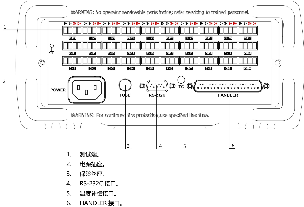
图 3-2 后面板
