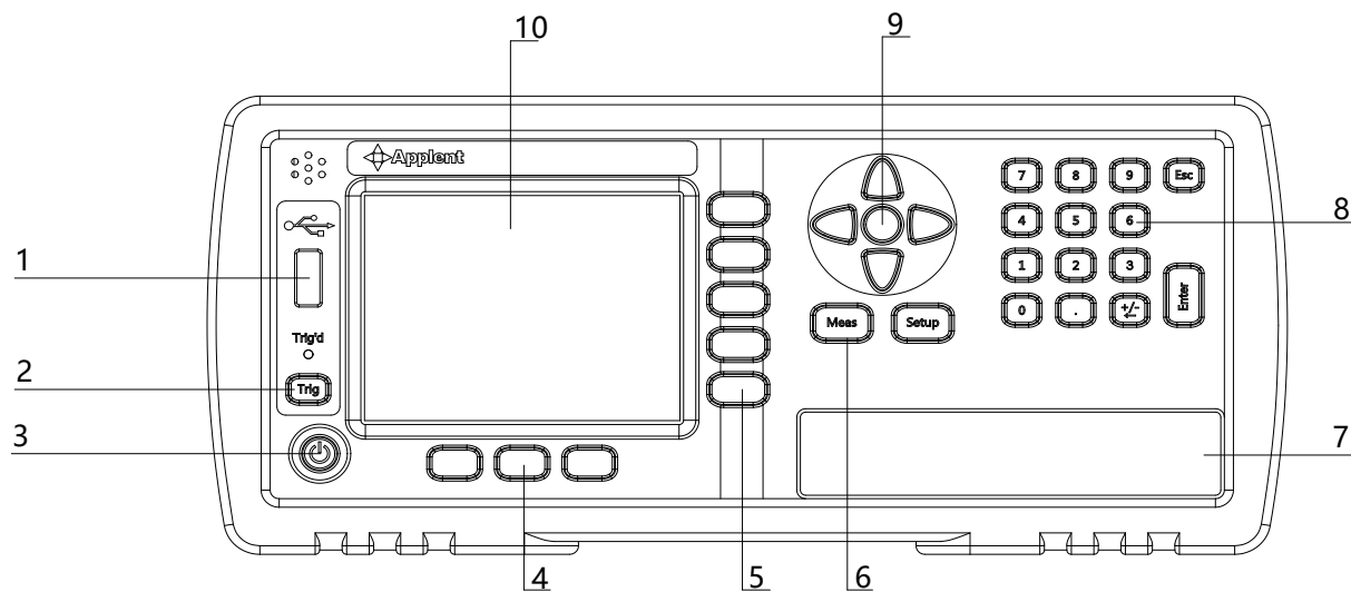
图 3-1 前面板
