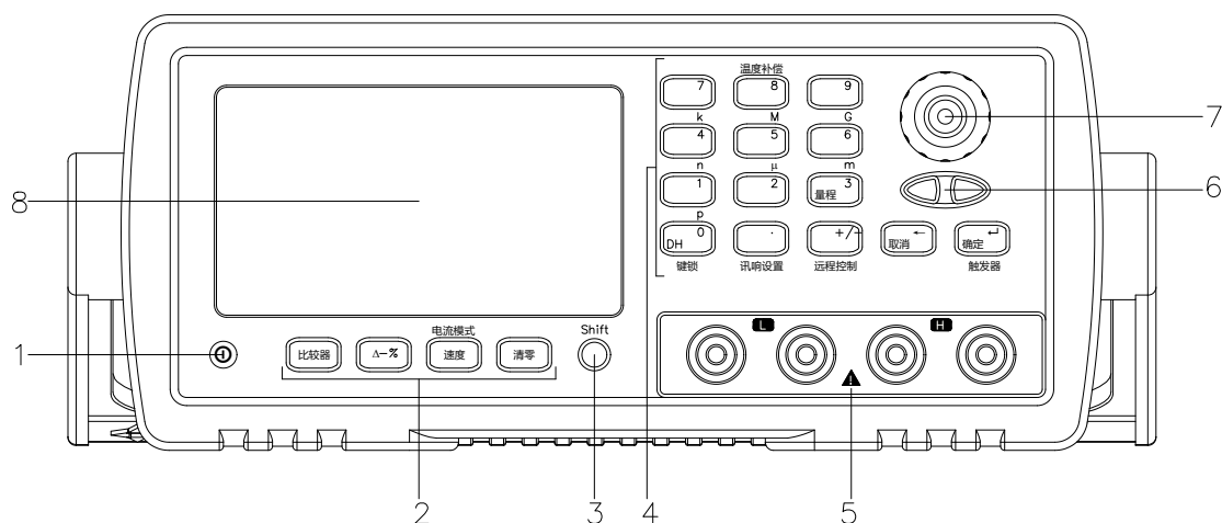
图 3-1 前面板
