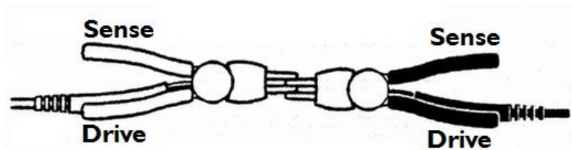
图 3-6 正确的测试端短路方法
