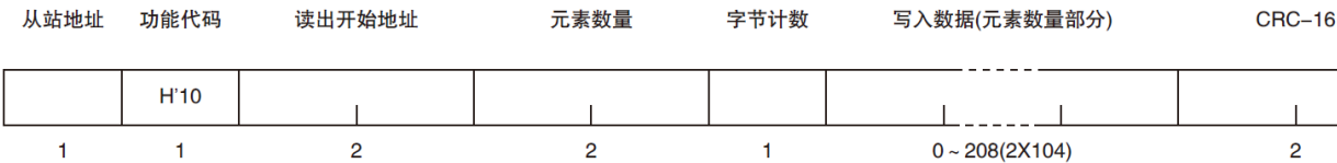
图 12-7 写入多个寄存器（0x10）
