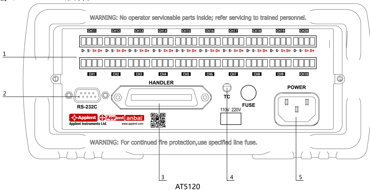
图 3-2 后面板
