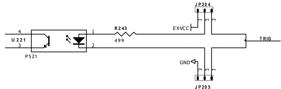
■ 输入端原理图 输入端原理图 (Trig)
