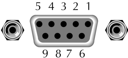
后面板上 RS-232 接口
