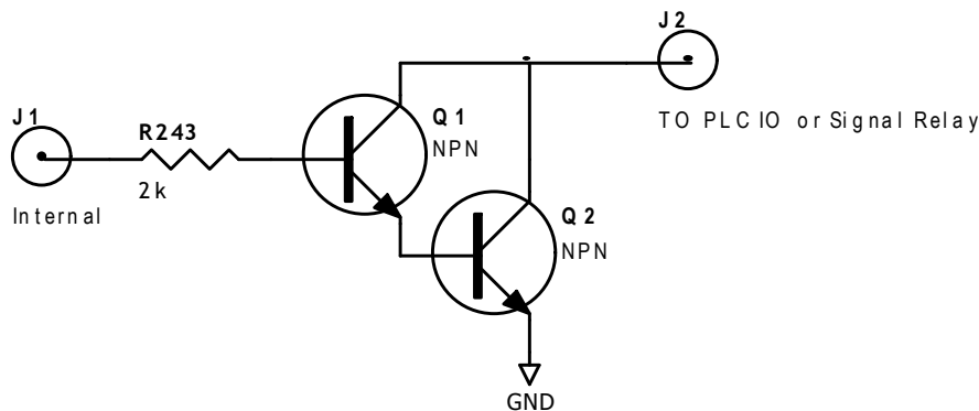
■ 输出端原理图 输出端原理图
