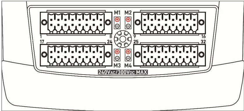
图 3-4 热电偶接线端
