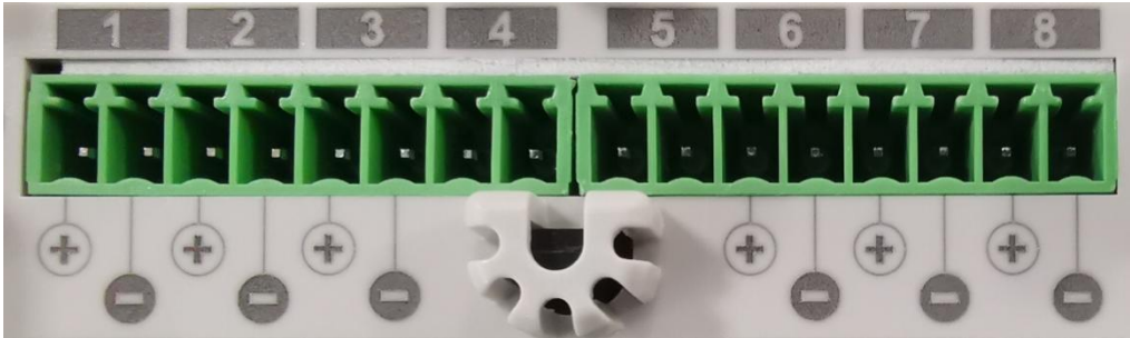
3- 3 接线端描述
