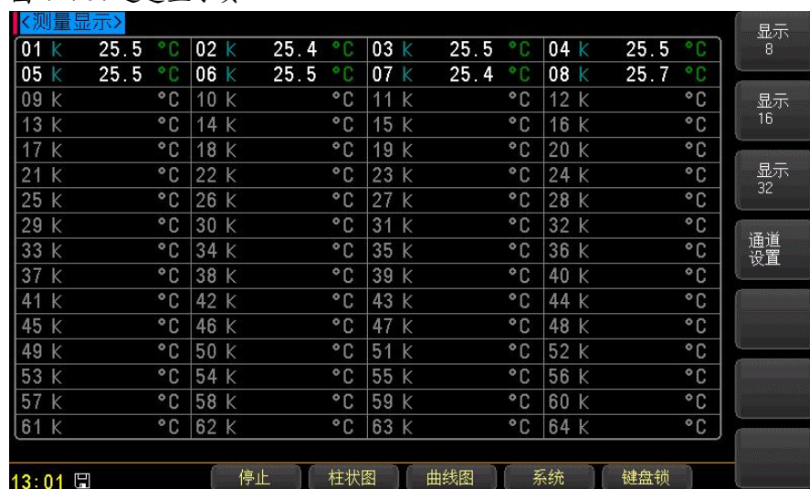
图 4-4 64 通道显示页
