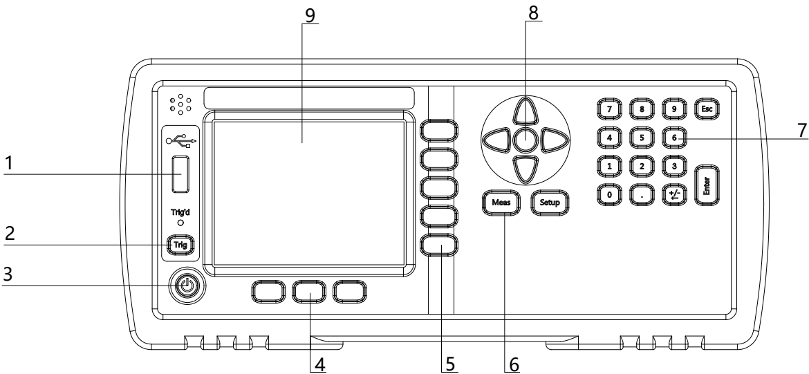
图 3- 1 前面板
