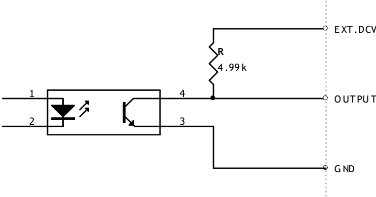
图 8-3 输出端原理图 输出端原理图 (分选, IDX, EOM)
