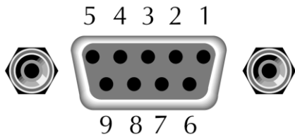
图 7-1 后面板上 RS-232 接口
