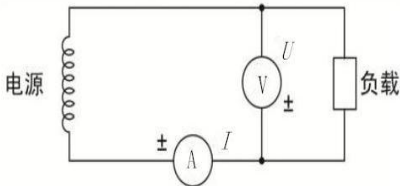
图 3-4 功率测量连接方法 2 — 将电压输入端子连接到负载侧的方法
