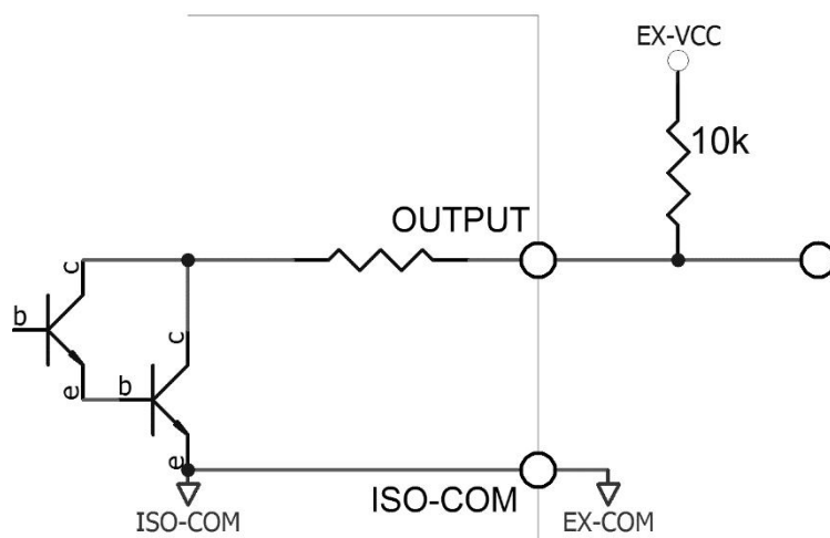
图 10-10 负逻辑输出
