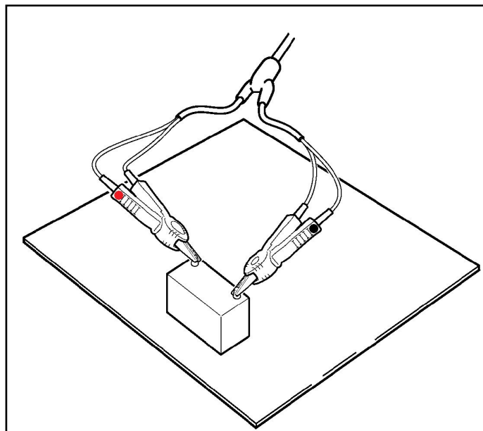
清零时务必注意位置要保持一致，在 30\text{m}\Omega 及以下量程尤其注意。 正确的短路方法
