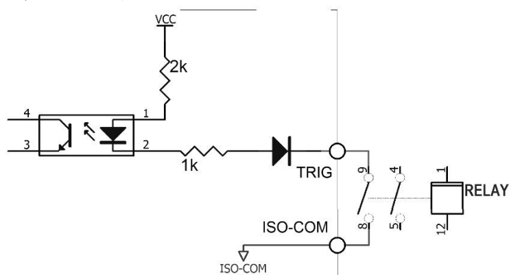
图 10-5 使用继电器控制
