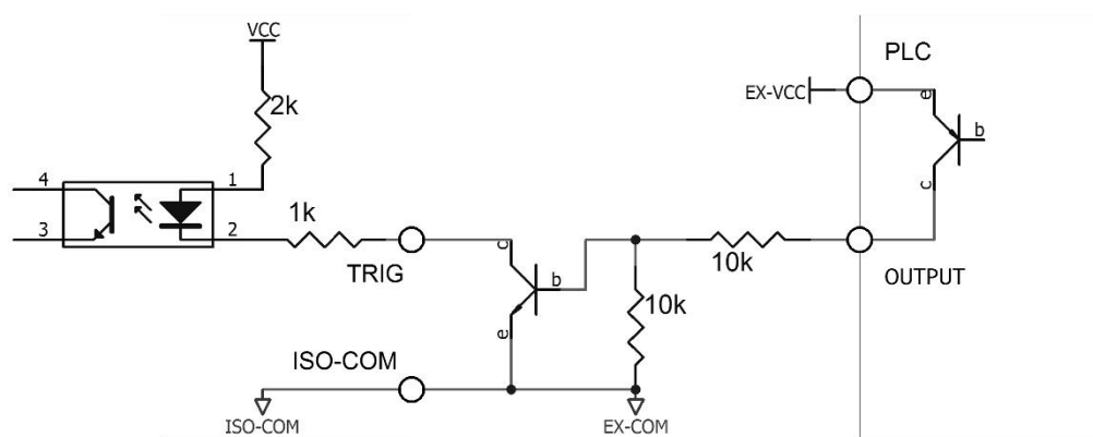
图 10-7 使用 PLC 正公共端子控制
