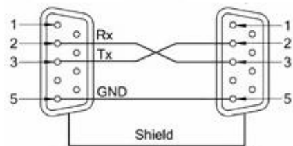
图 11-2 后面板上 RS-232 接口[公头]
