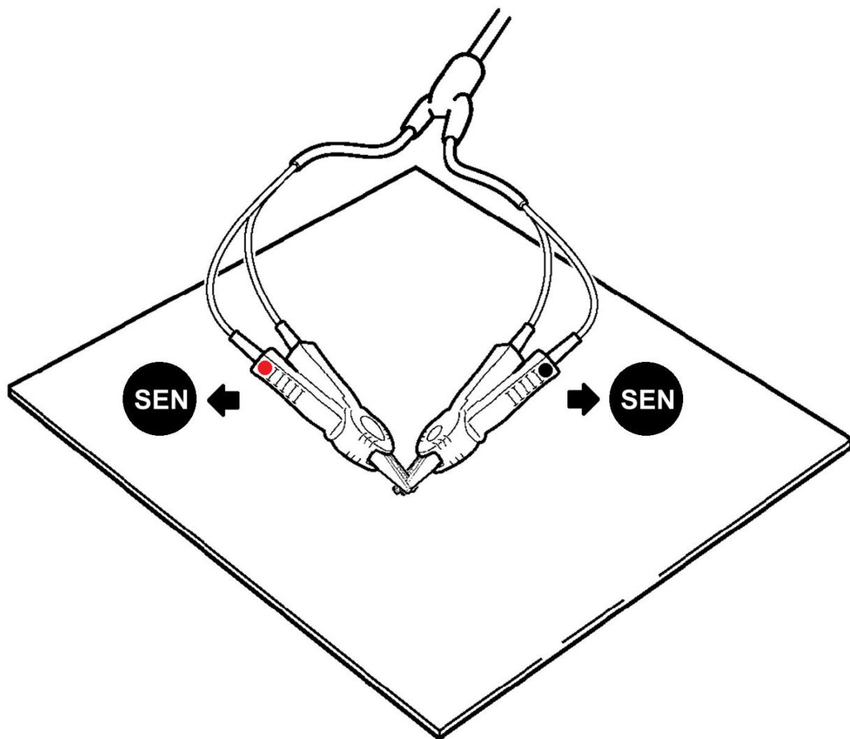
清零时务必注意位置要保持一致，在 30\text{m}\Omega 及以下量程尤其注意。 正确的短路方法
