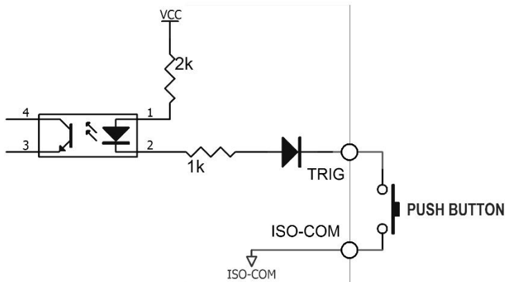
图 10-4 与开关的连接
