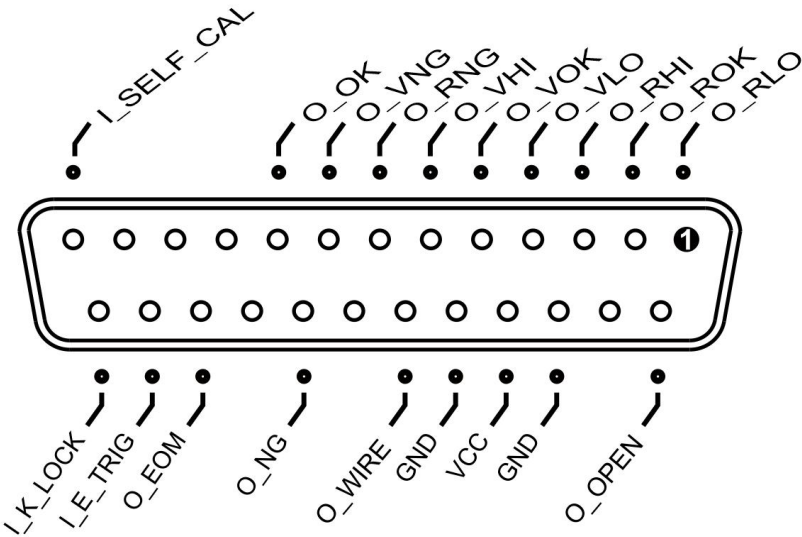
■ 输出端（所有信号都为低有效） 输出端引脚定义
