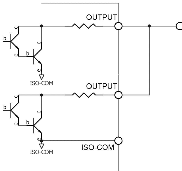
图 10-12 输出到 PLC 负公共端子
