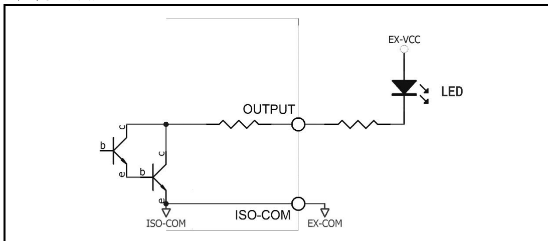
图 8-9 控制发光二极管或光电耦合器
