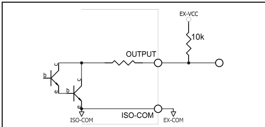
图 8-11 双端口输出组成逻辑或电路
